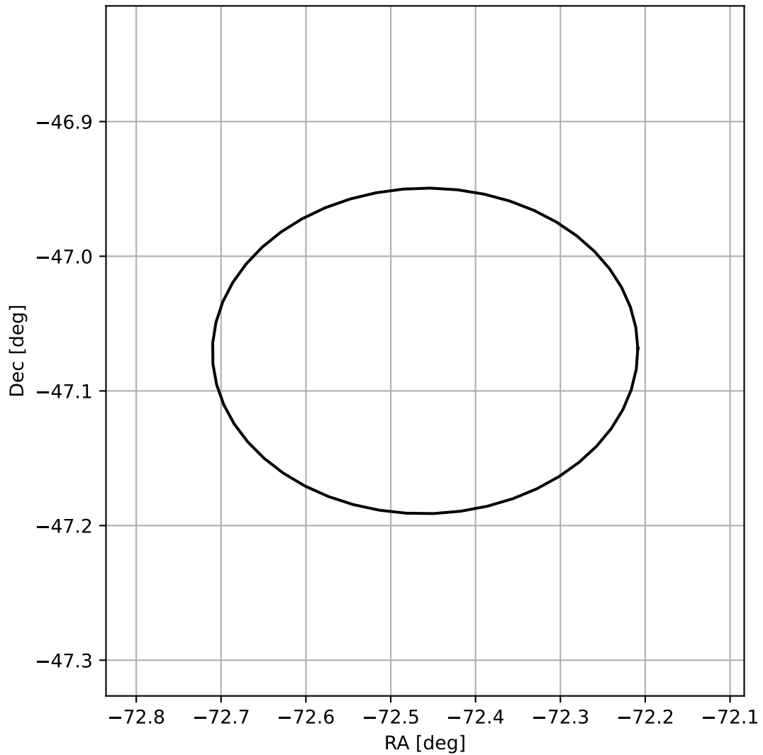
4FGL J1910.1-4704
