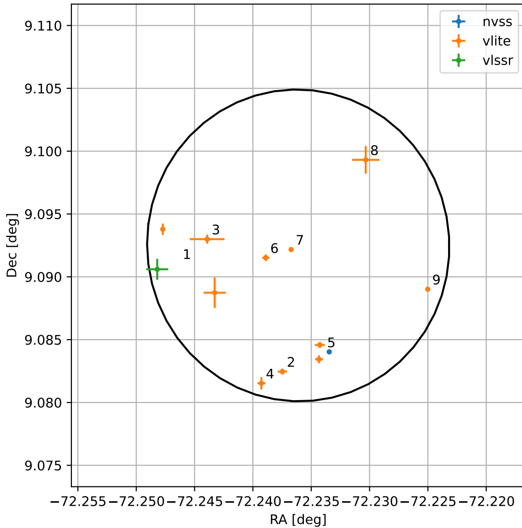
4FGL J1911.0+0905
