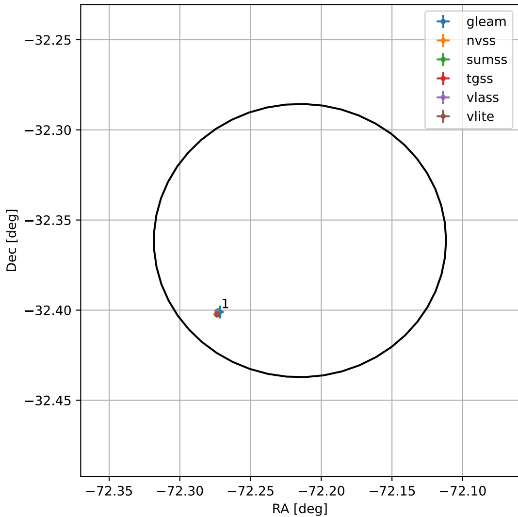
4FGL J1911.1-3221
