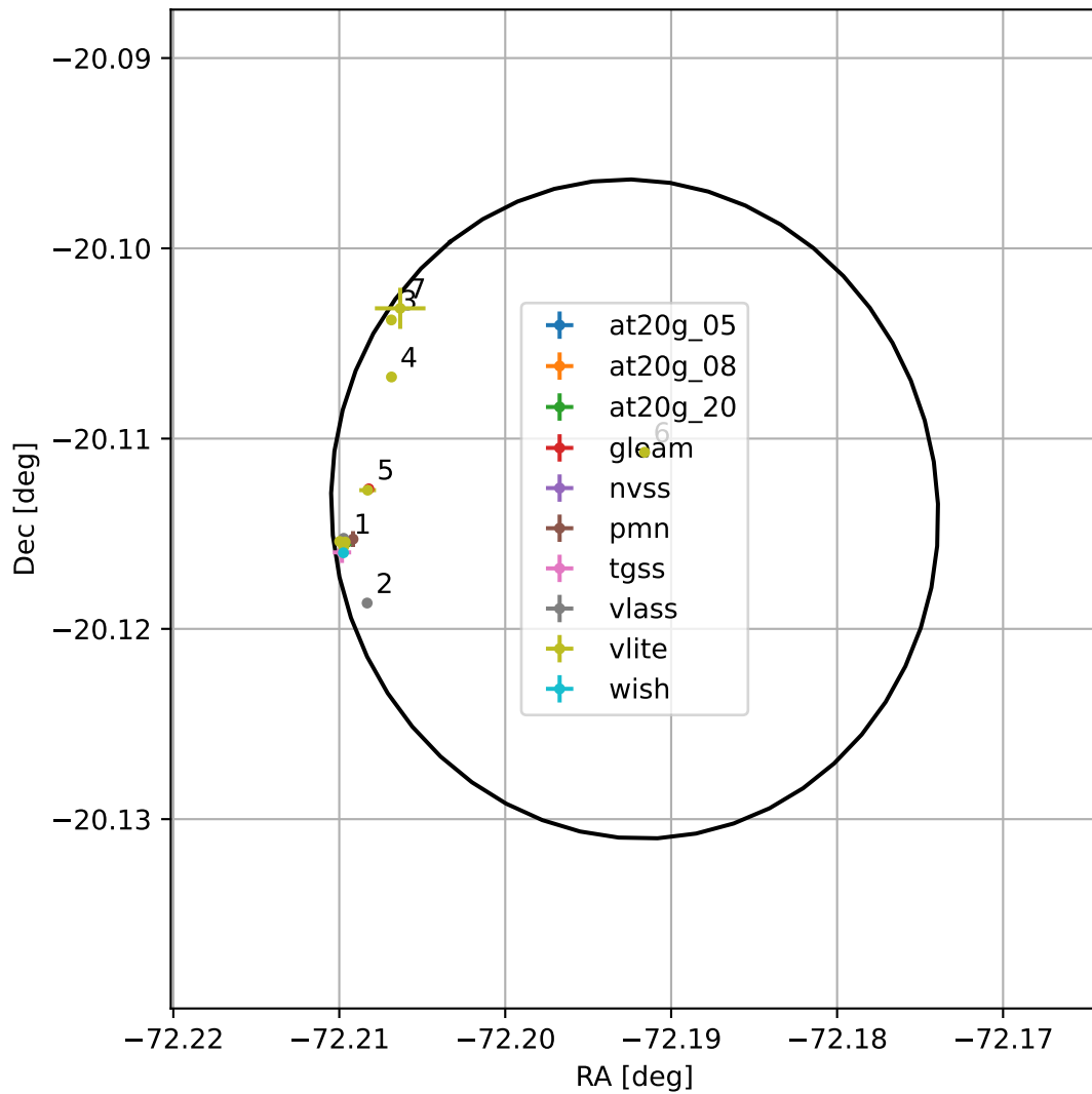
4FGL J1911.2-2006
