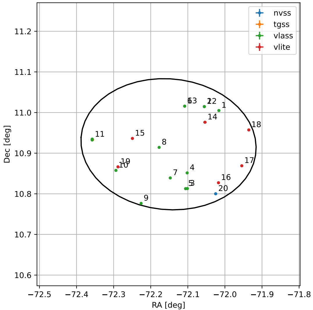
4FGL J1911.3+1055
