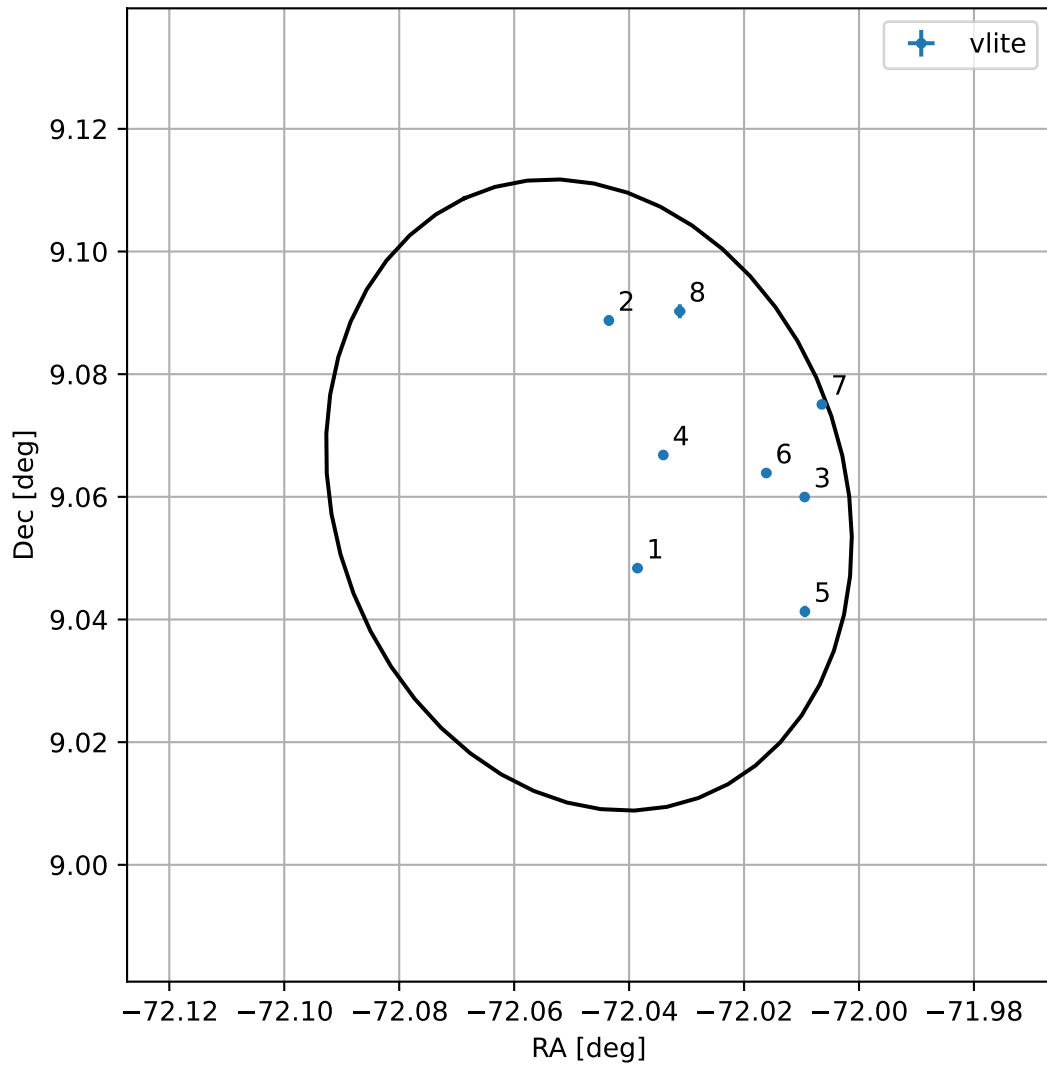
4FGL J1911.8+0903
