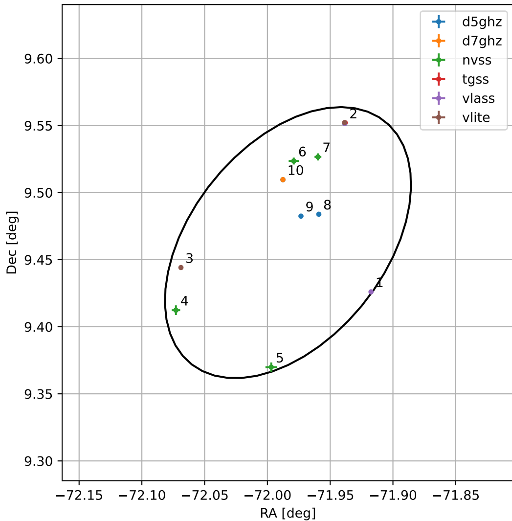
4FGL J1912.0+0927
