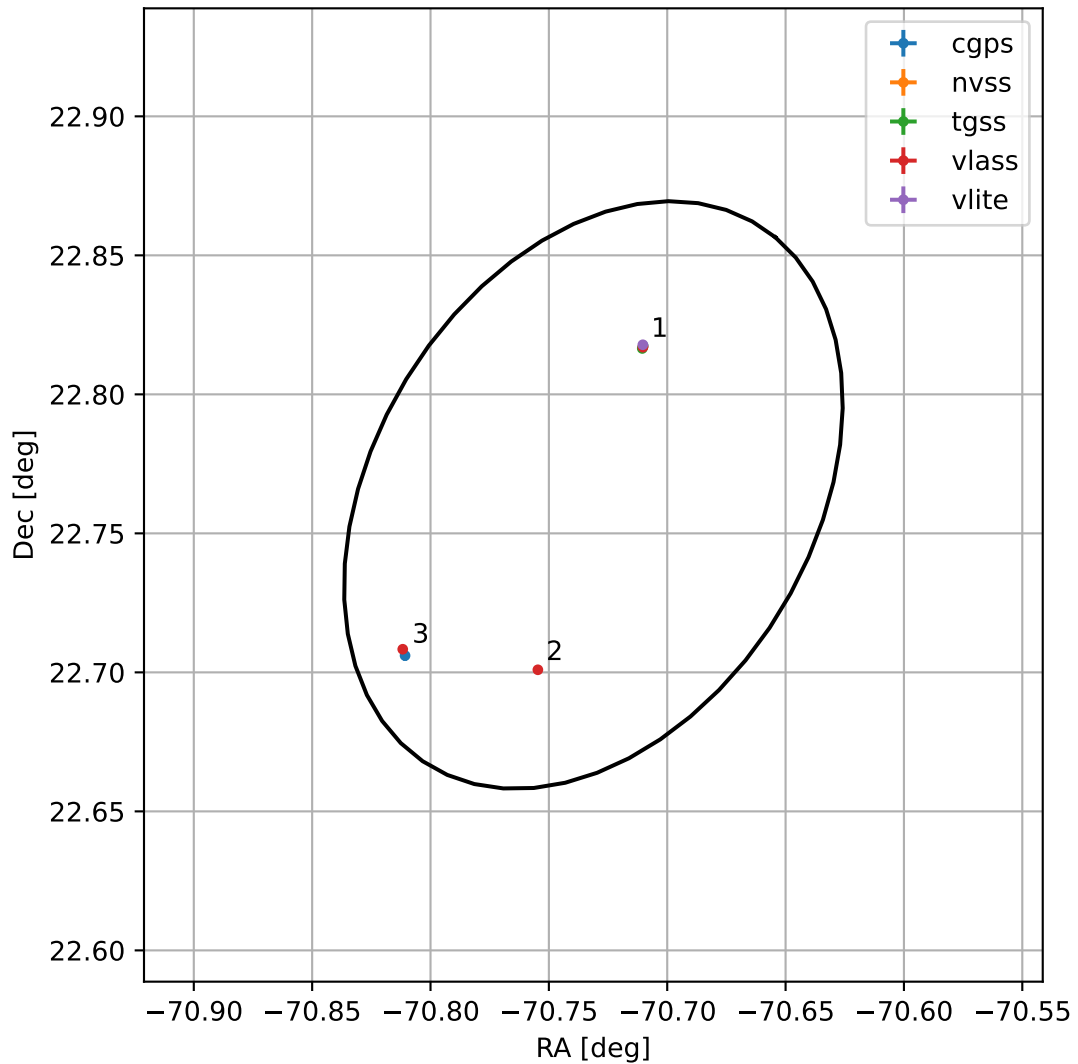
4FGL J1917.0+2245
