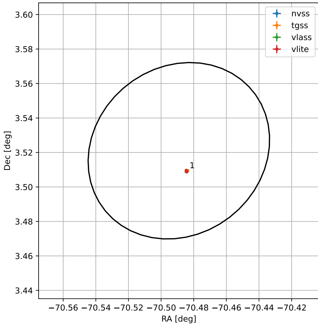
4FGL J1918.0+0331
