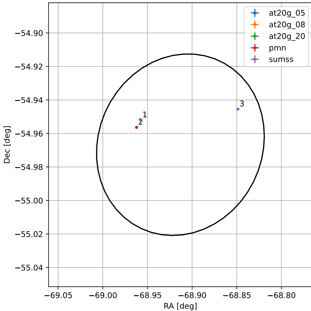
4FGL J1924.3-5458
