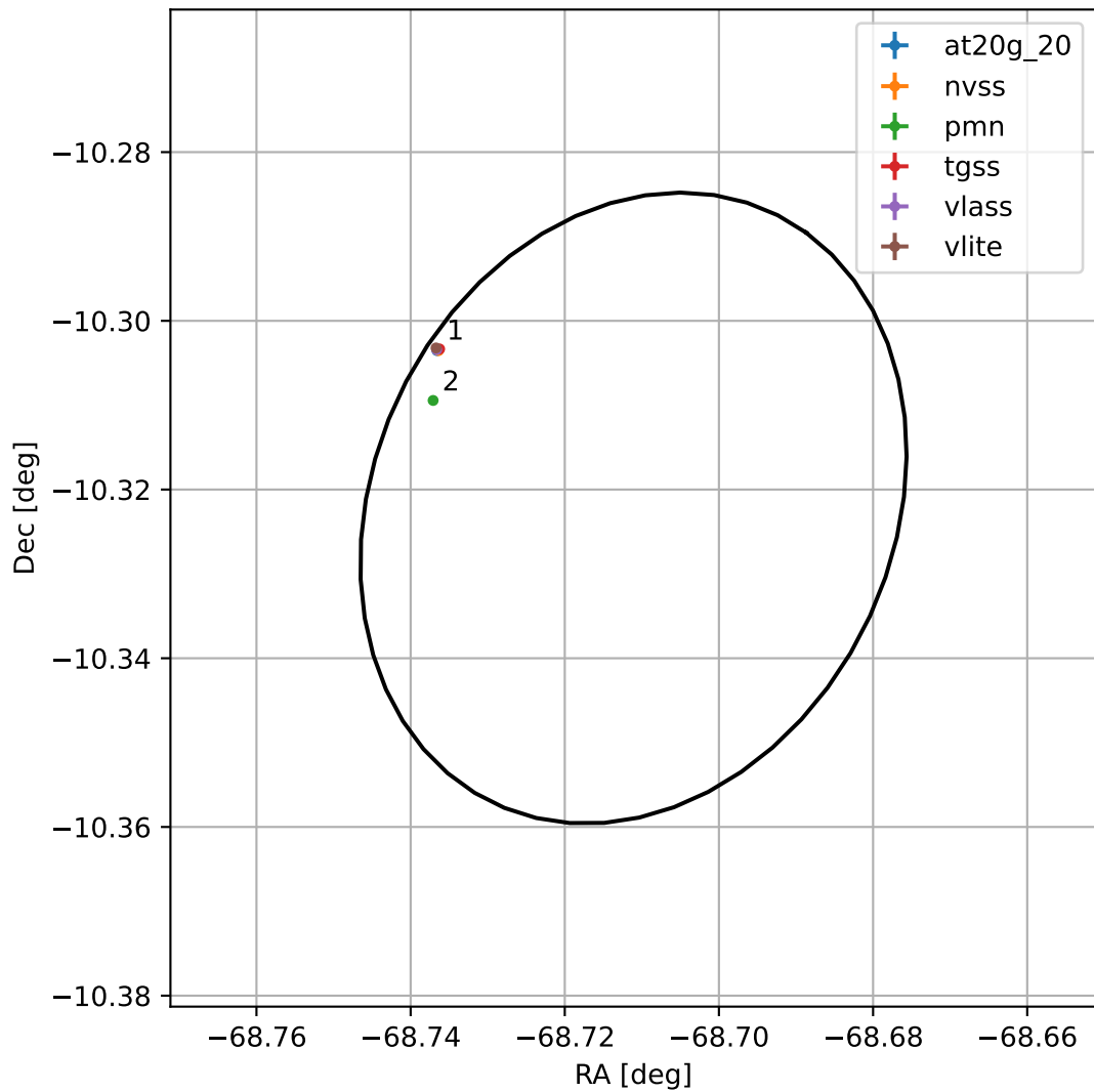
4FGL J1925.1-1019
