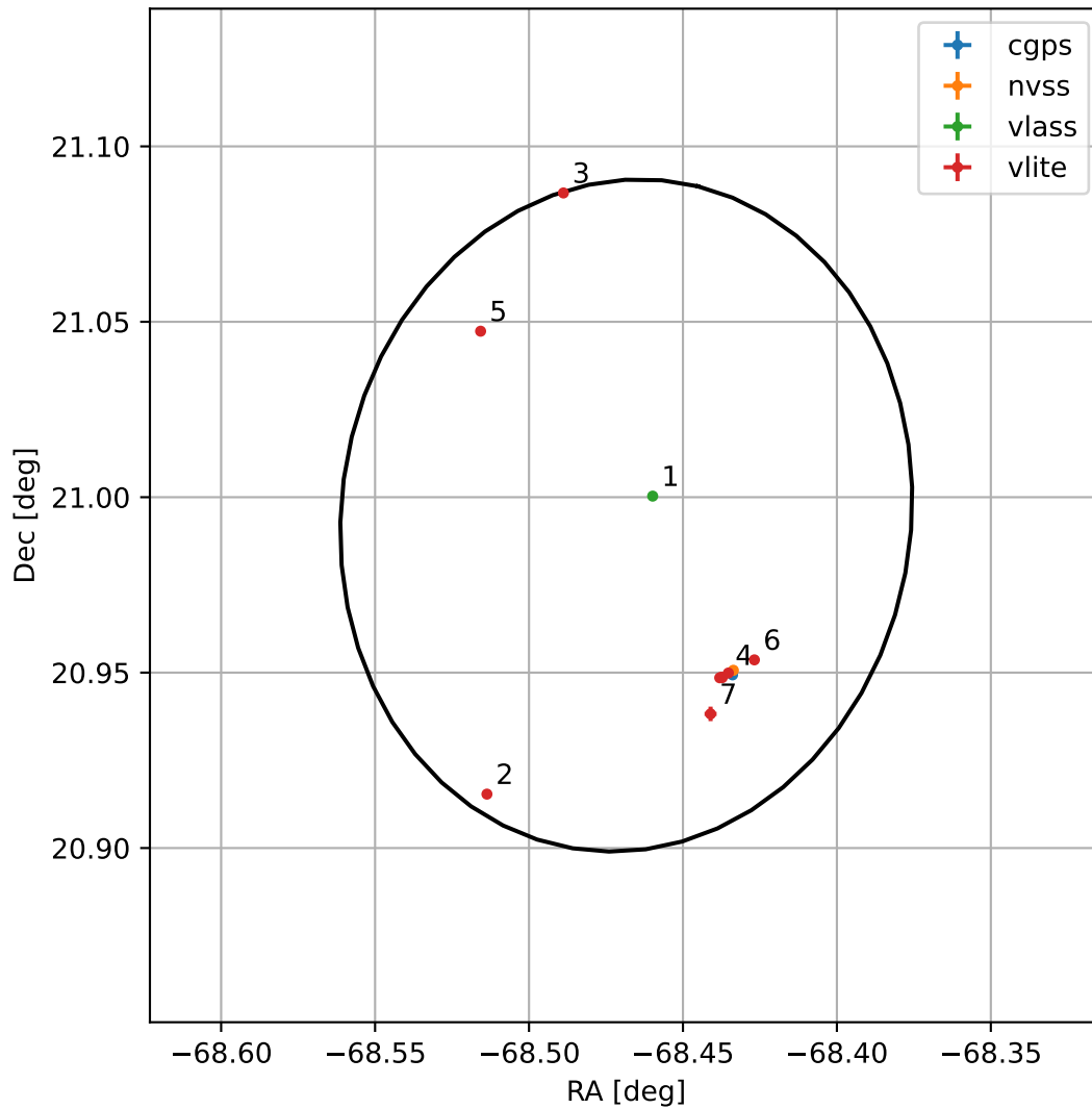
4FGL J1926.1+2059
