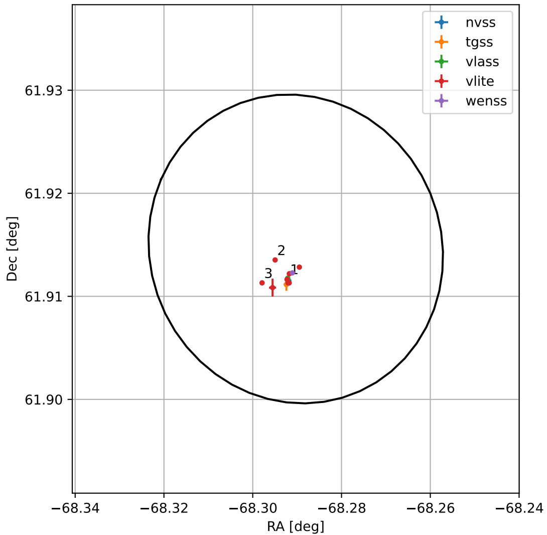
4FGL J1926.8+6154
