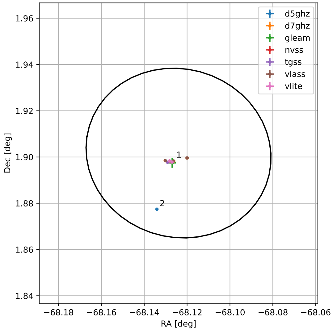
4FGL J1927.5+0154
