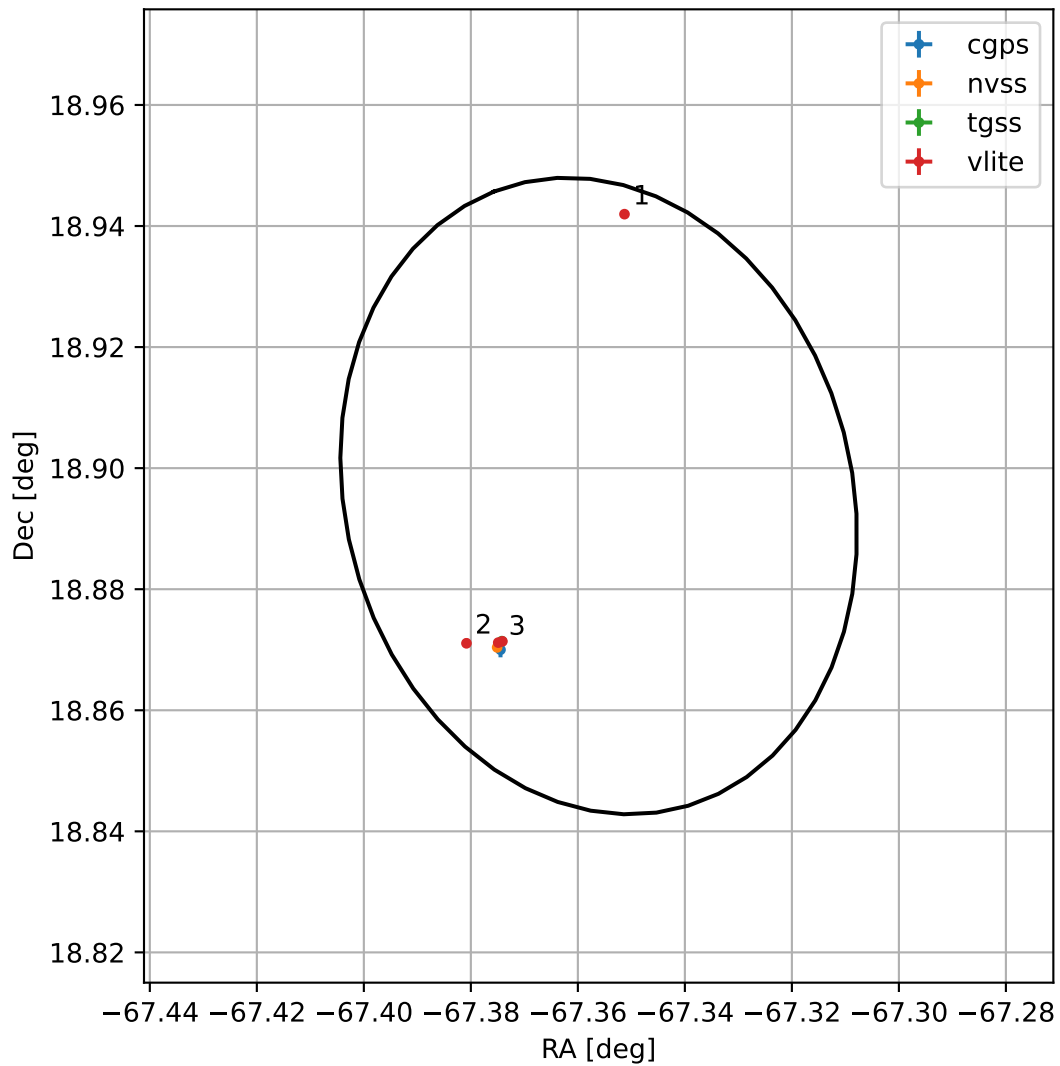
4FGL J1930.5+1853
