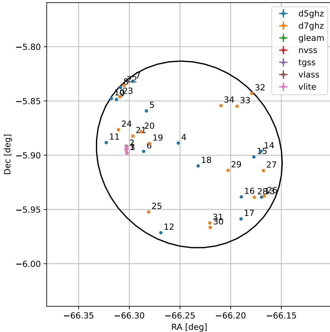
4FGL J1935.0-0553
