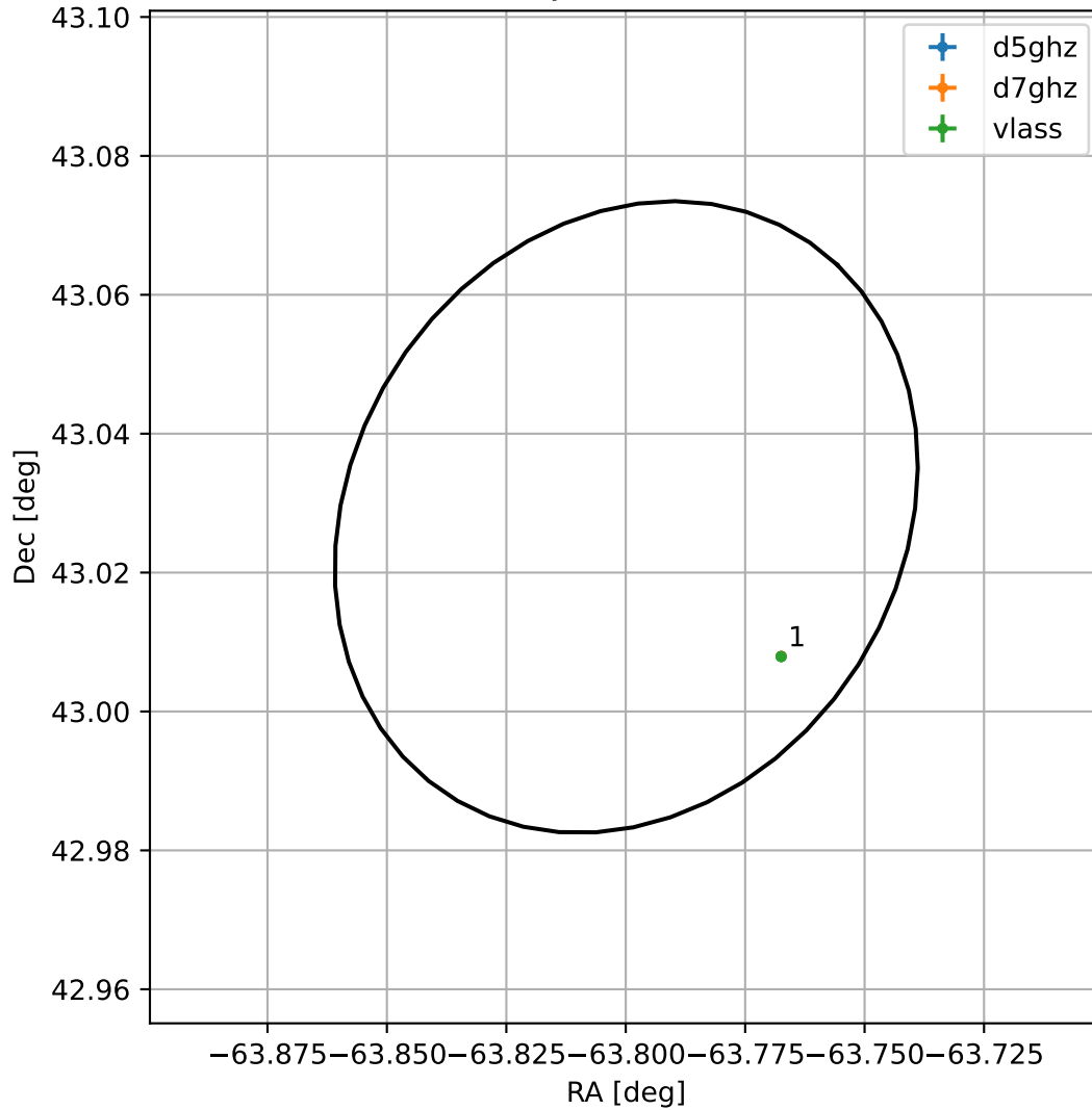
4FGL J1944.8+4301
