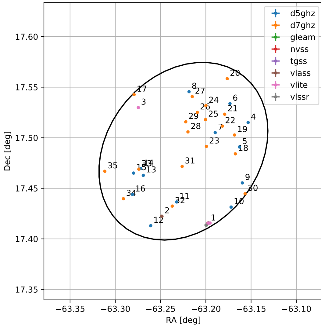
4FGL J1947.1+1729
