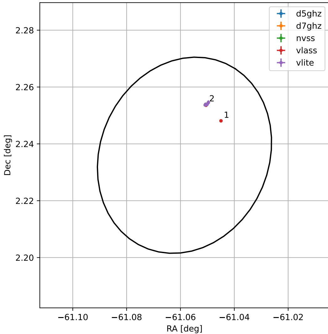
4FGL J1955.7+0214
