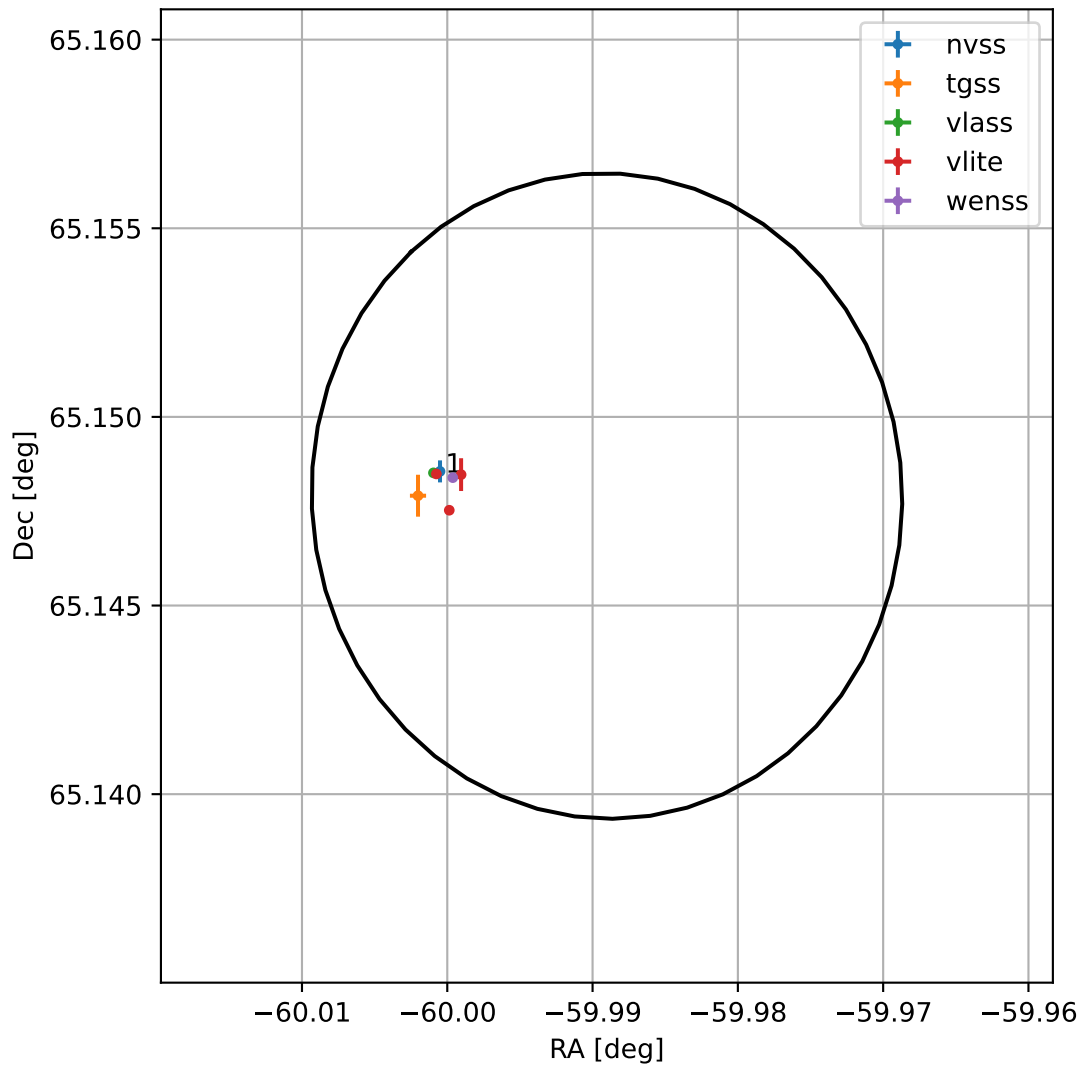
4FGL J2000.0+6508
