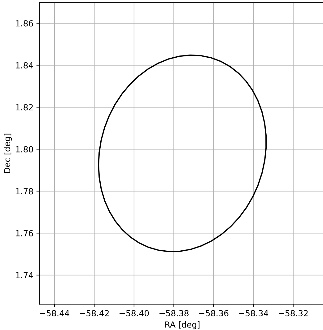
4FGL J2006.4+0147
