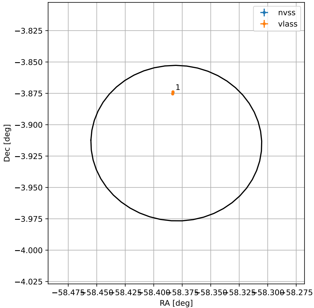
4FGL J2006.4-0354
