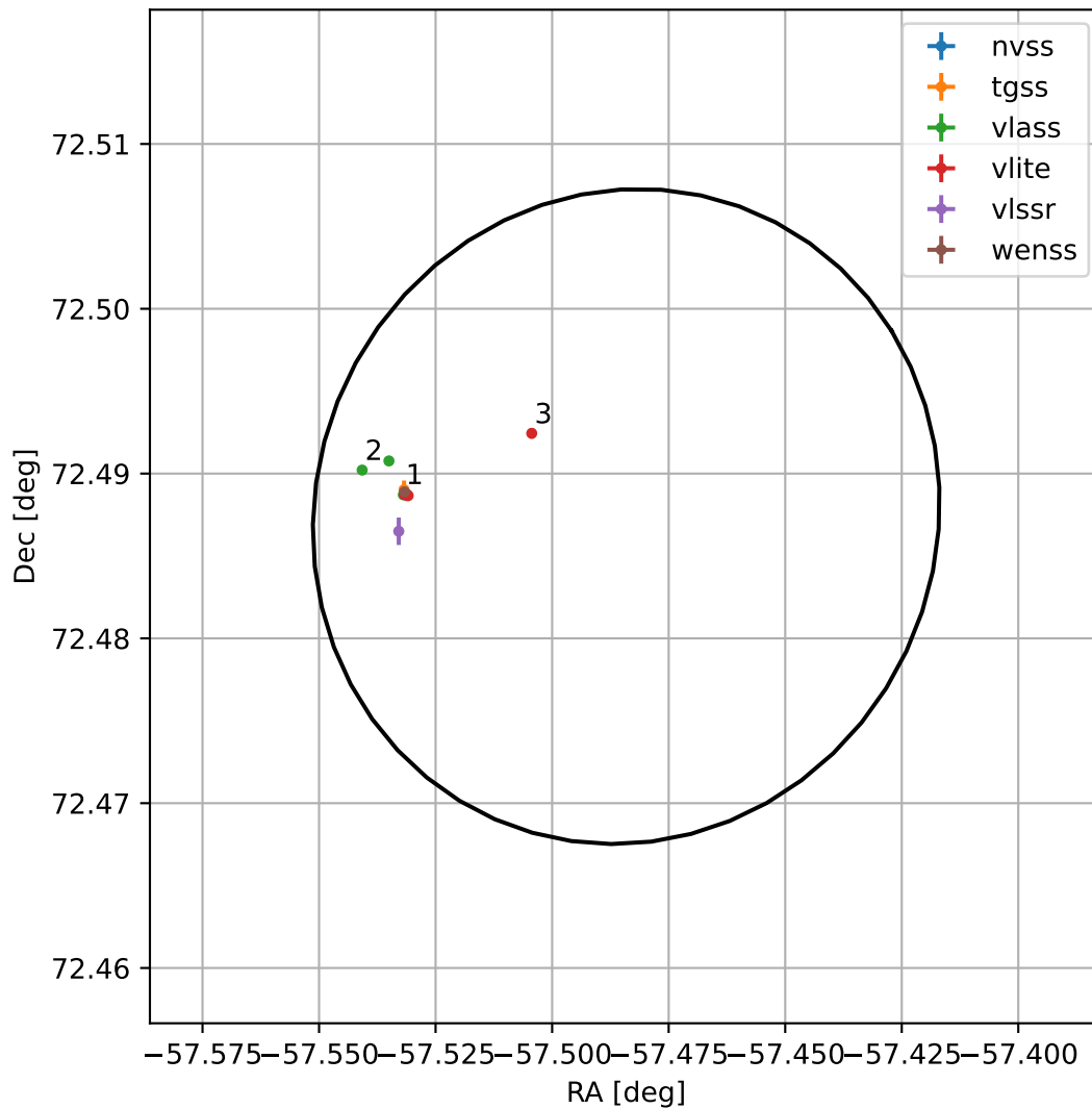
4FGL J2010.0+7229
