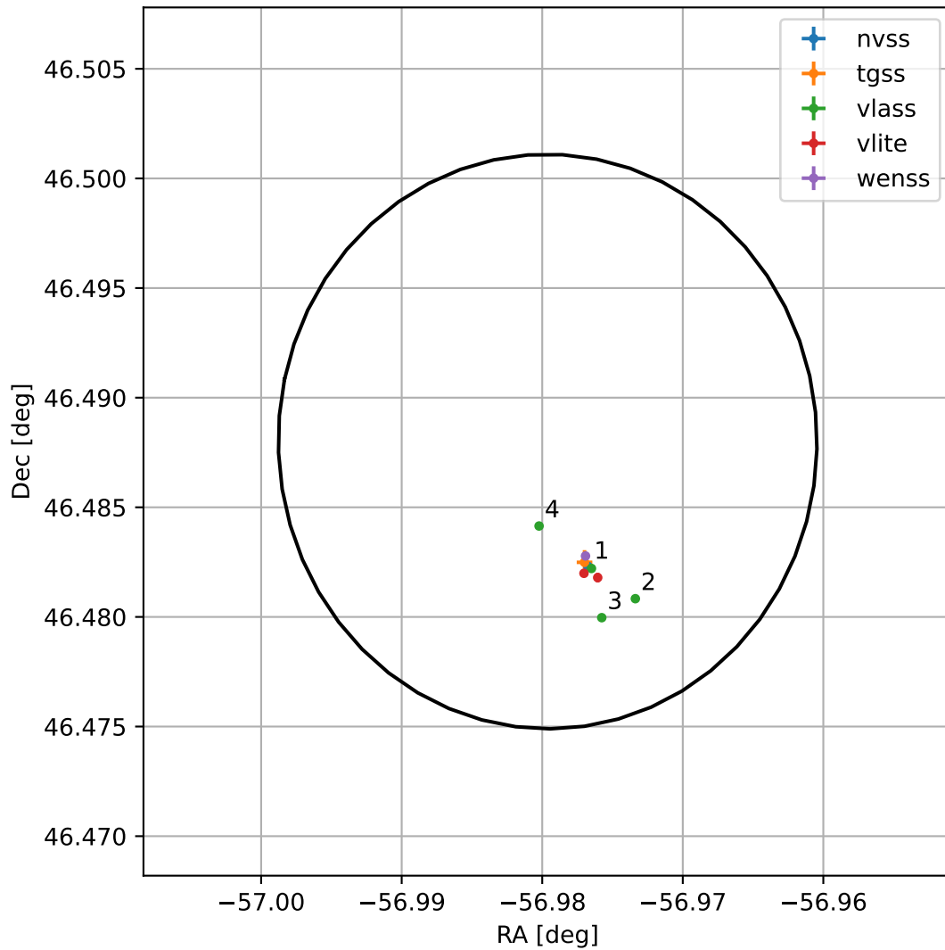
4FGL J2012.0+4629
