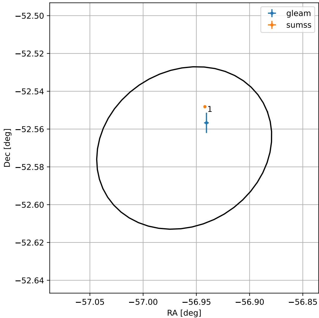
4FGL J2012.1-5234
