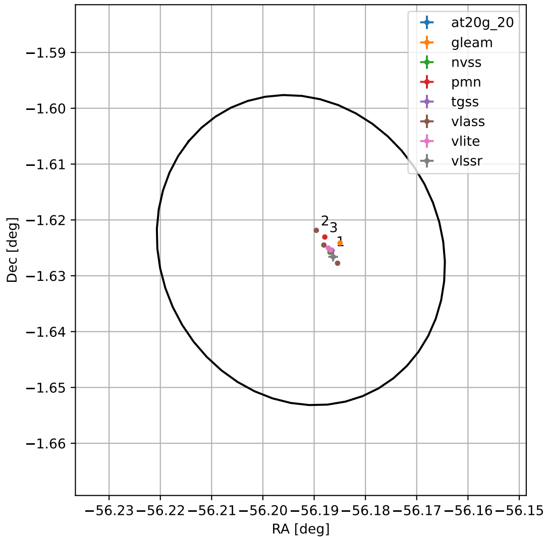
4FGL J2015.2-0137
