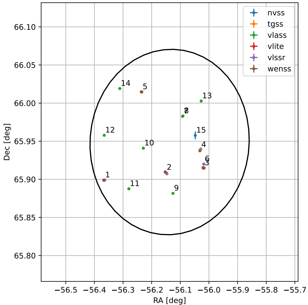
4FGL J2015.4+6556
