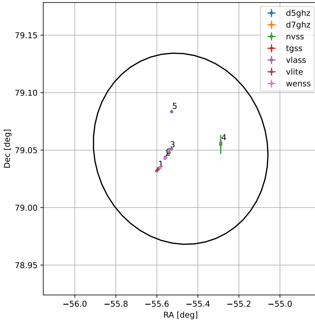
4FGL J2018.0+7903
