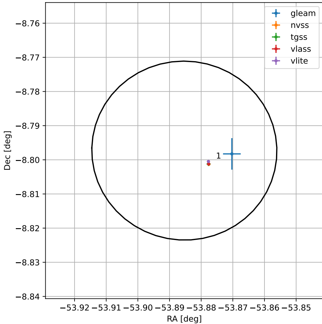
4FGL J2024.4-0847
