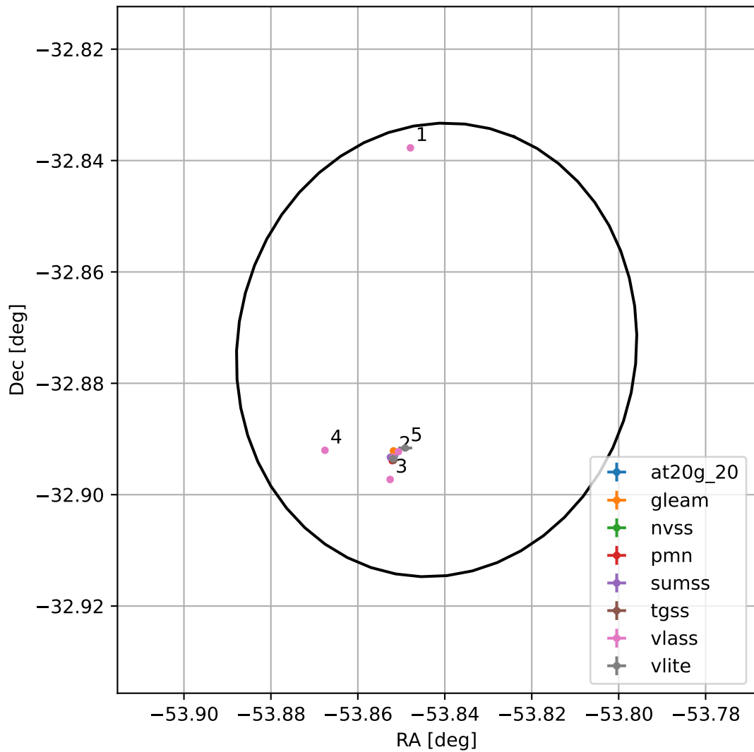
4FGL J2024.6-3252
