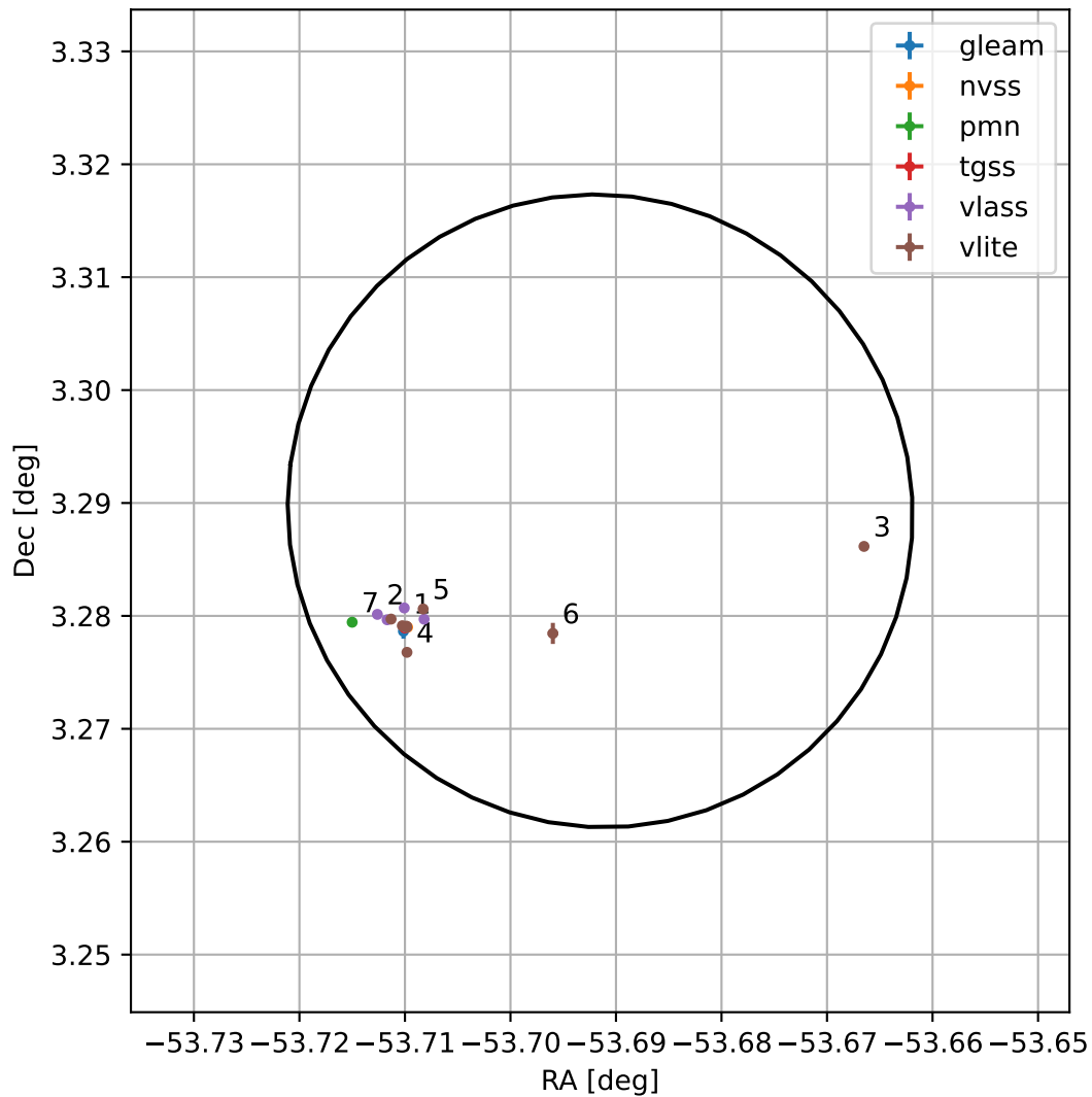
4FGL J2025.2+0317
