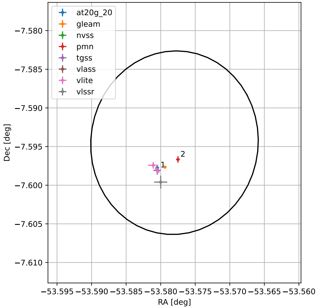
4FGL J2025.6-0735
