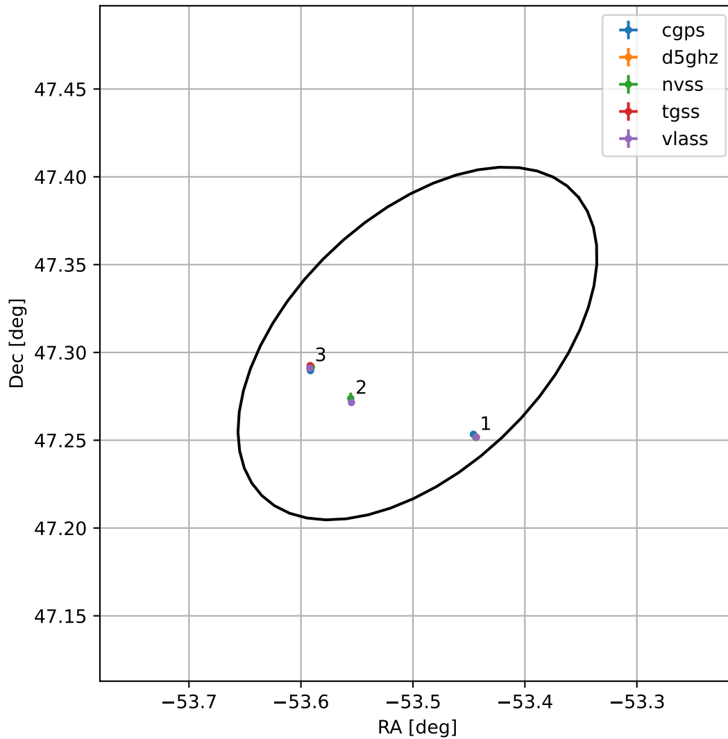
4FGL J2026.0+4718
