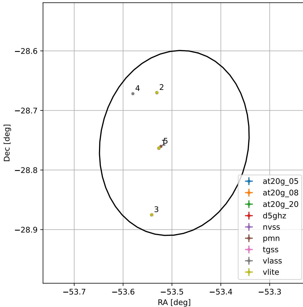
4FGL J2026.0-2845
