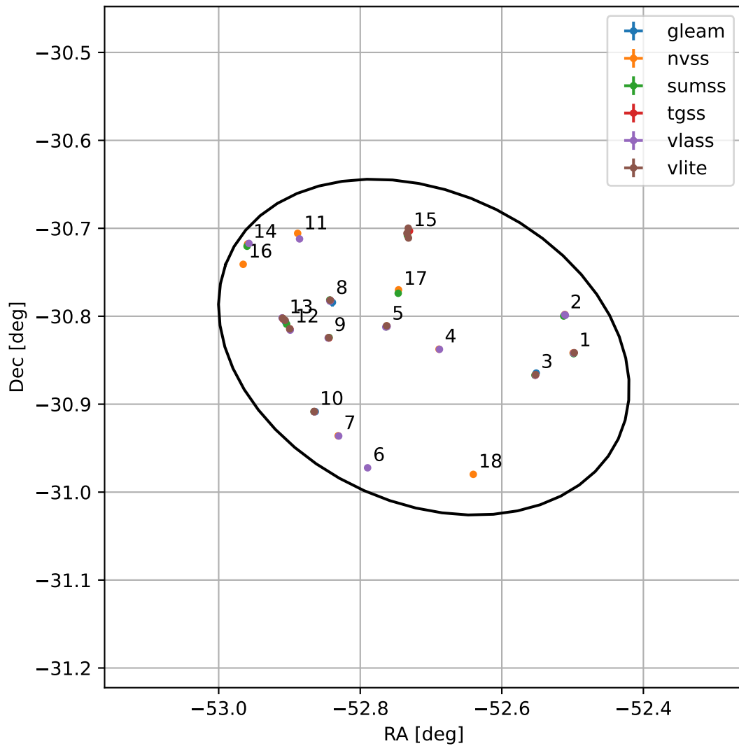
4FGL J2029.1-3050
