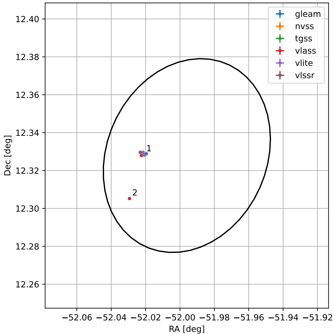
4FGL J2032.0+1219
