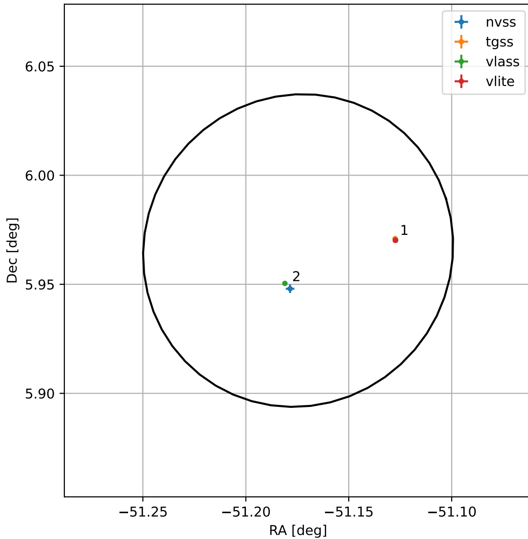
4FGL J2035.3+0557
