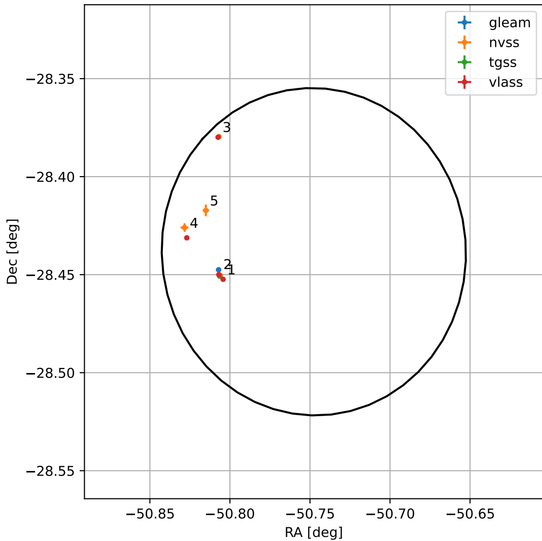
4FGL J2037.0-2826
