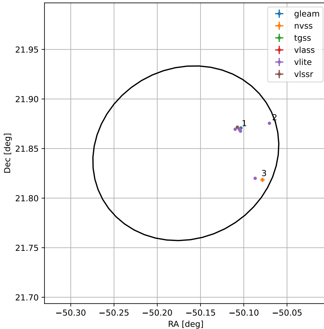
4FGL J2039.3+2150
