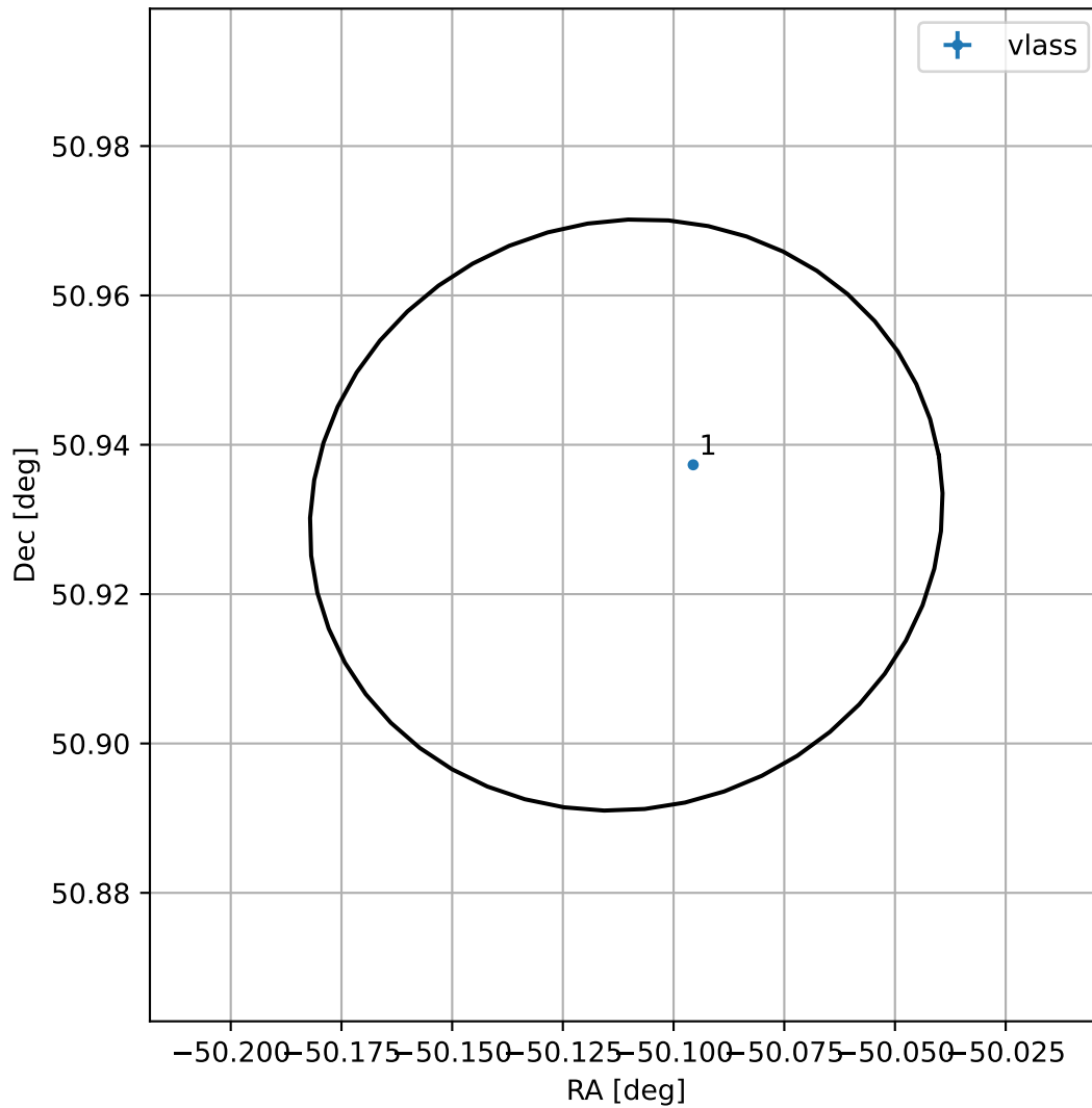
4FGL J2039.5+5055
