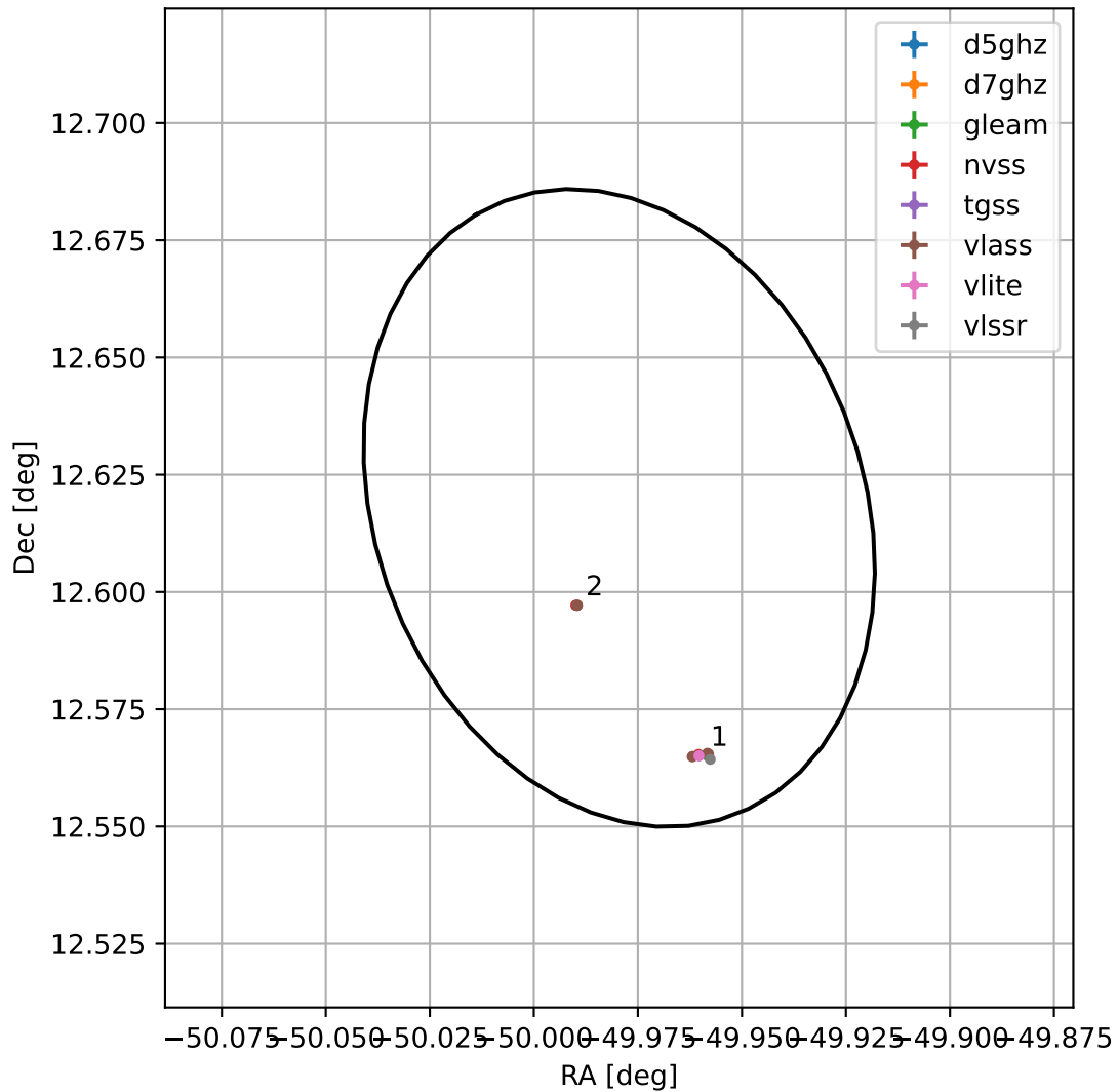
4FGL J2040.0+1237
