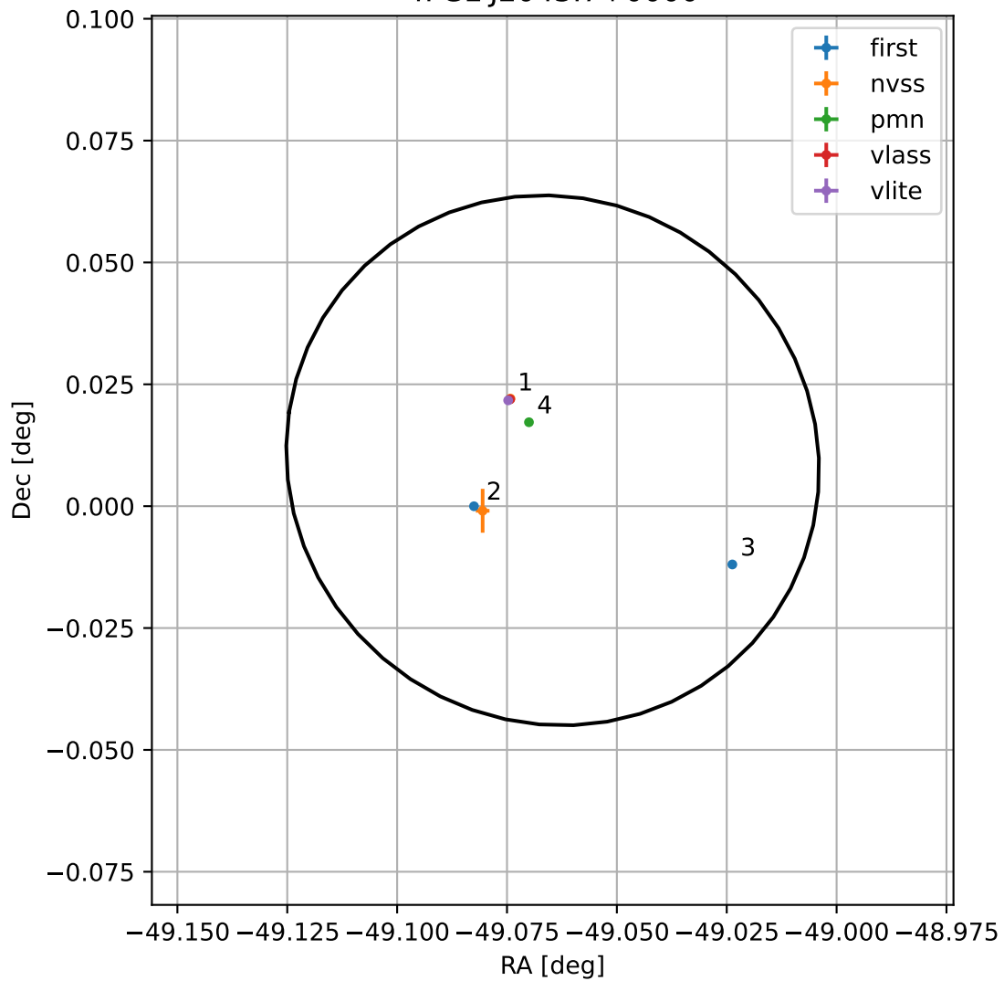
4FGL J2043.7+0000
