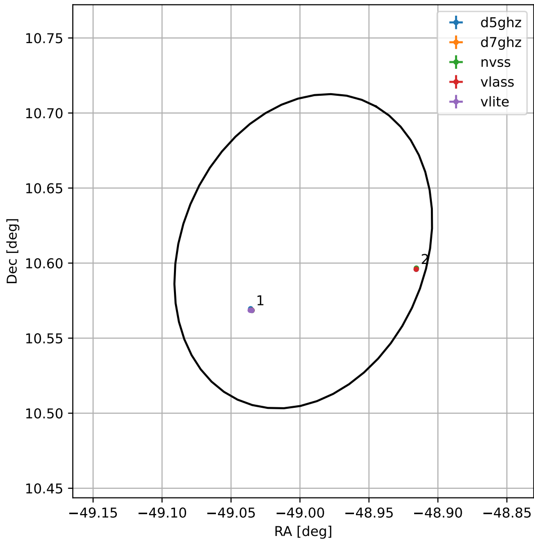
4FGL J2044.0+1036
