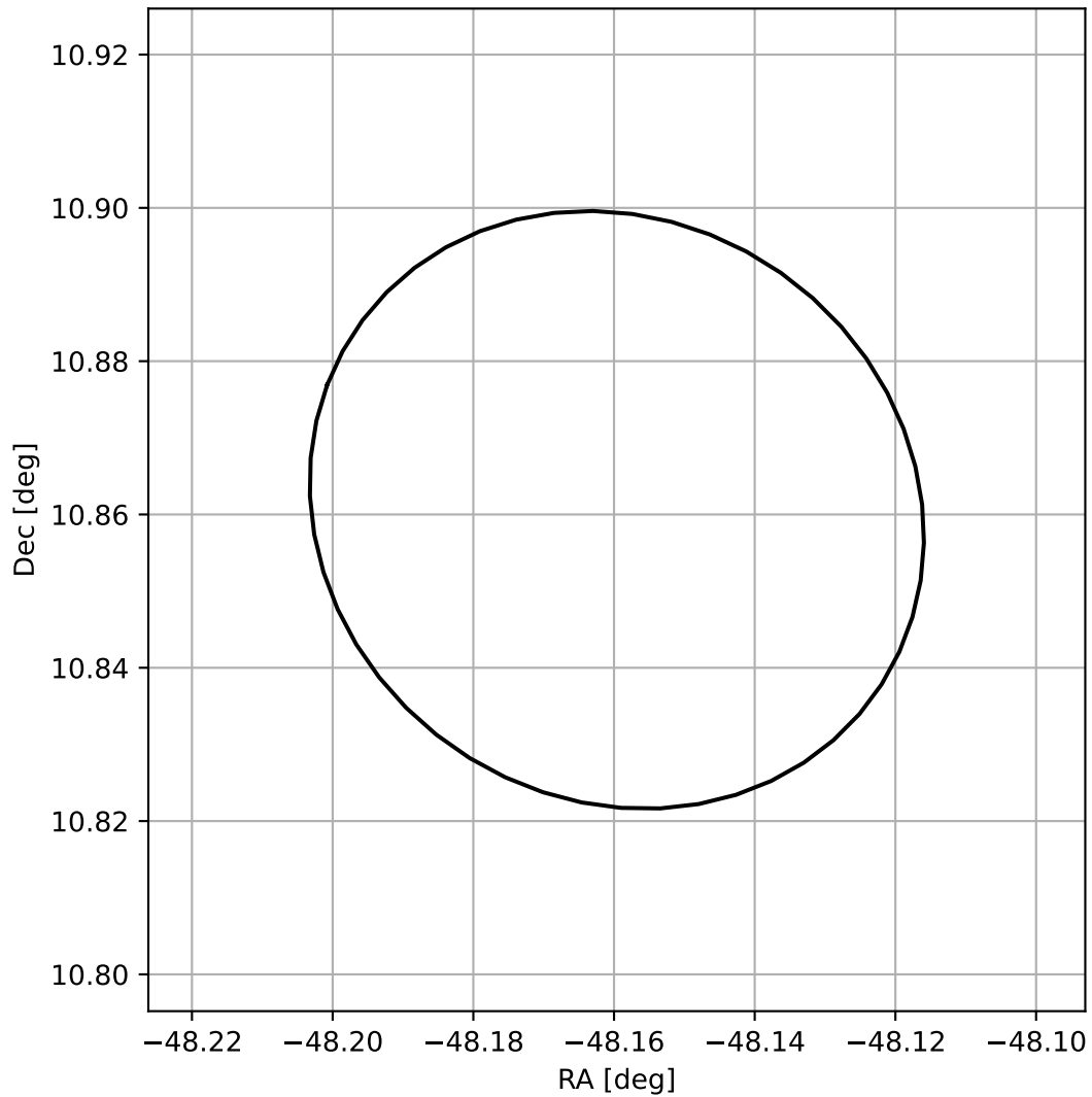
4FGL J2047.3+1051
