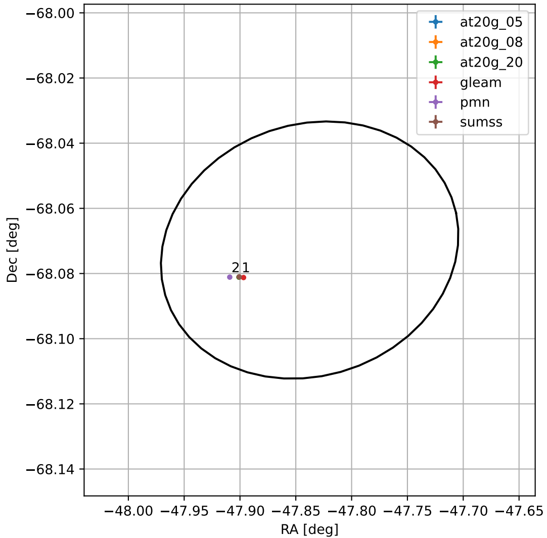
4FGL J2048.6-6804
