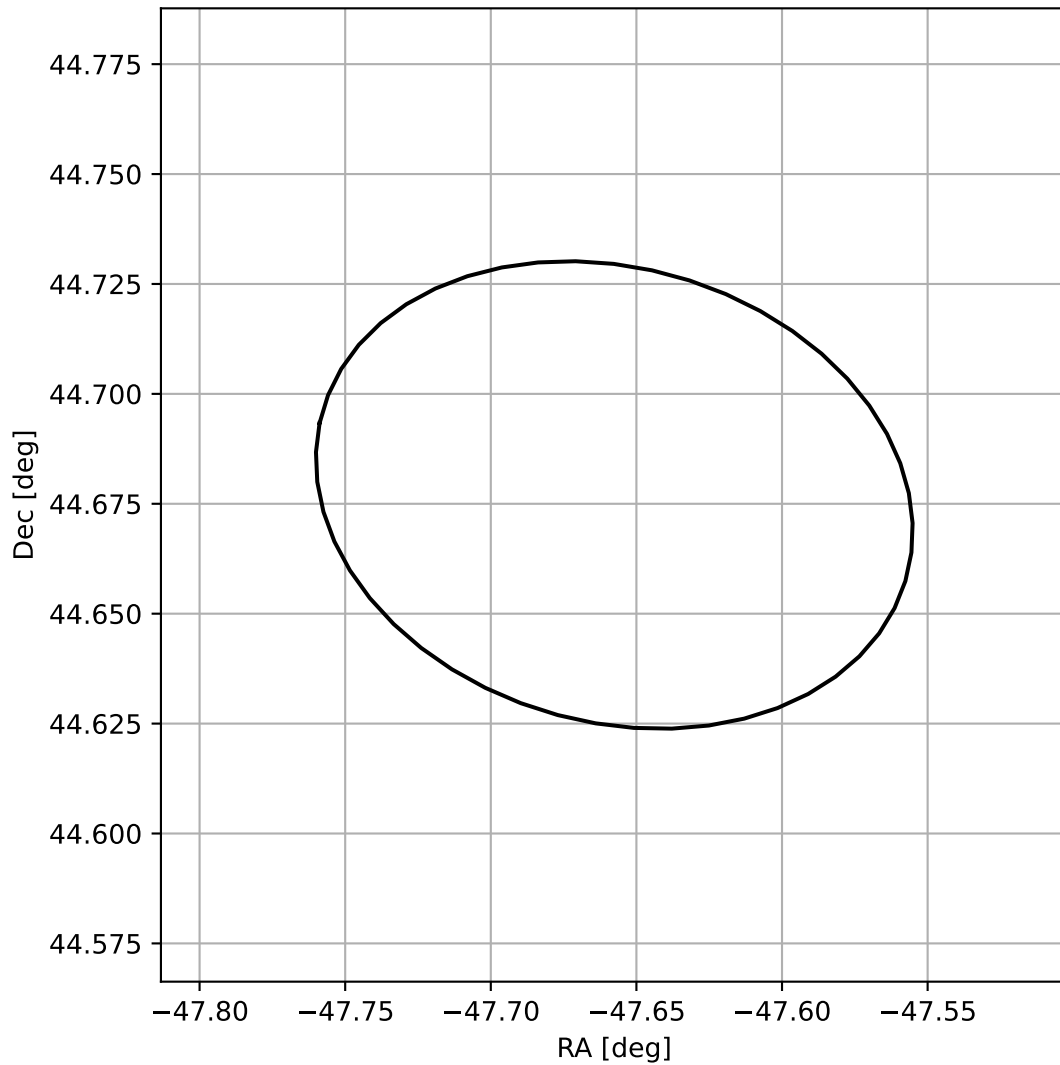
4FGL J2049.3+4440
