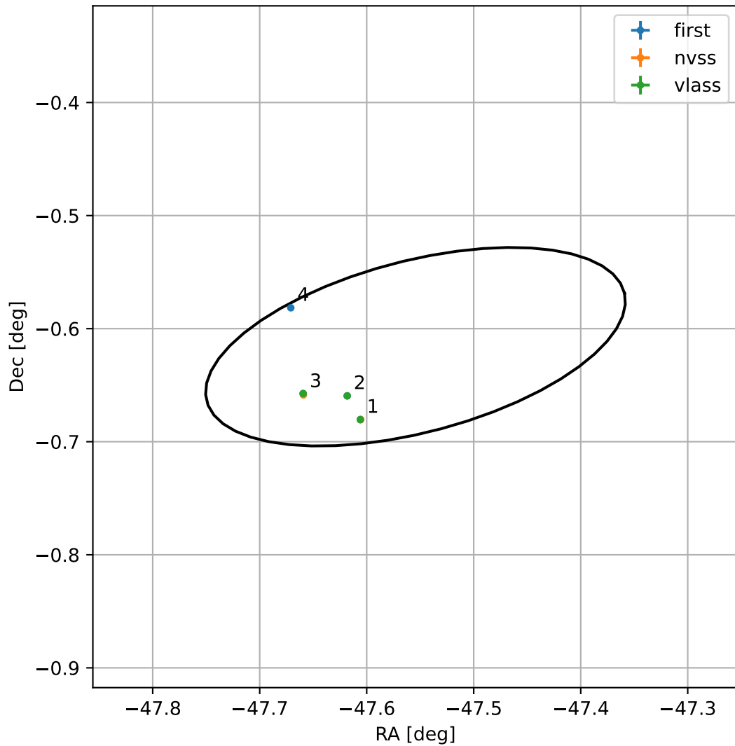
4FGL J2049.7-0036
