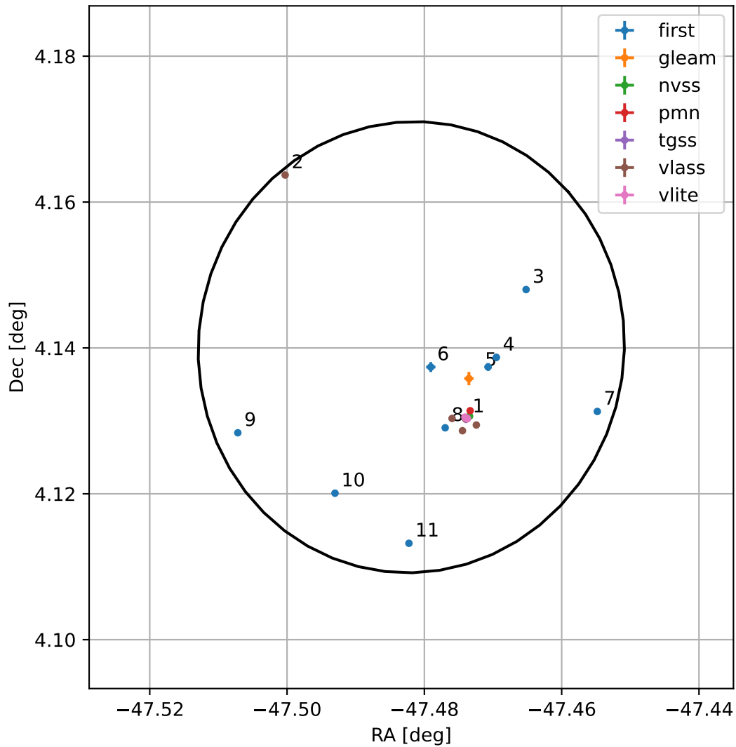
4FGL J2050.0+0408
