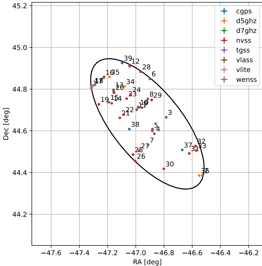
4FGL J2052.3+4437
