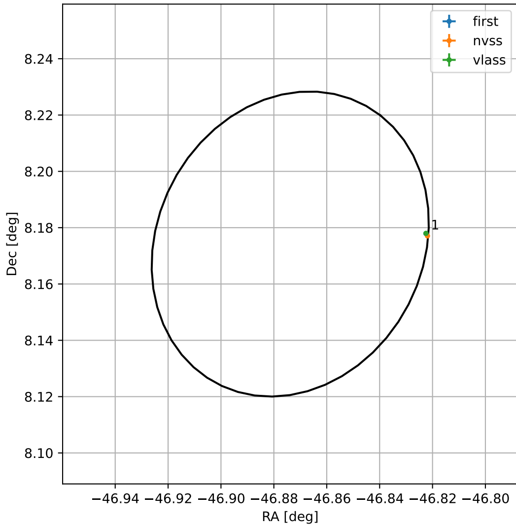
4FGL J2052.5+0810
